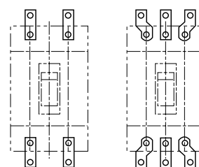
[ 2 pole ]
