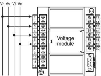
3P4W wiring
