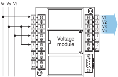
3P3W wiring
